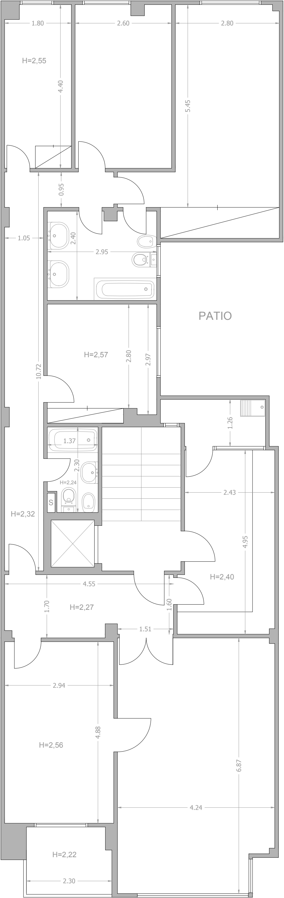
PLANO ESTADO ACTUAL (COTAS)
