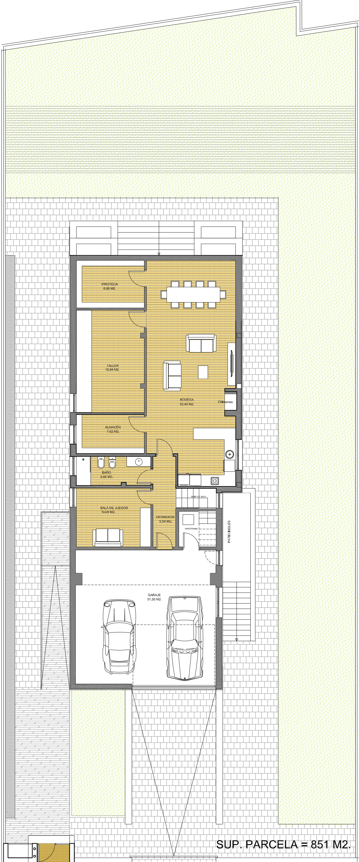
PLANTA SÓTANO
